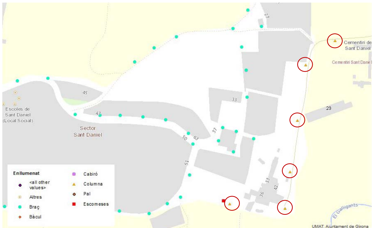
Esquema d'Enllumenat públic
