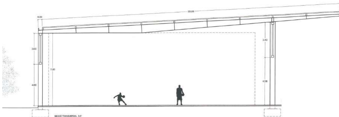
Secció d'una proposta equivalent de coberta de pista esportiva
