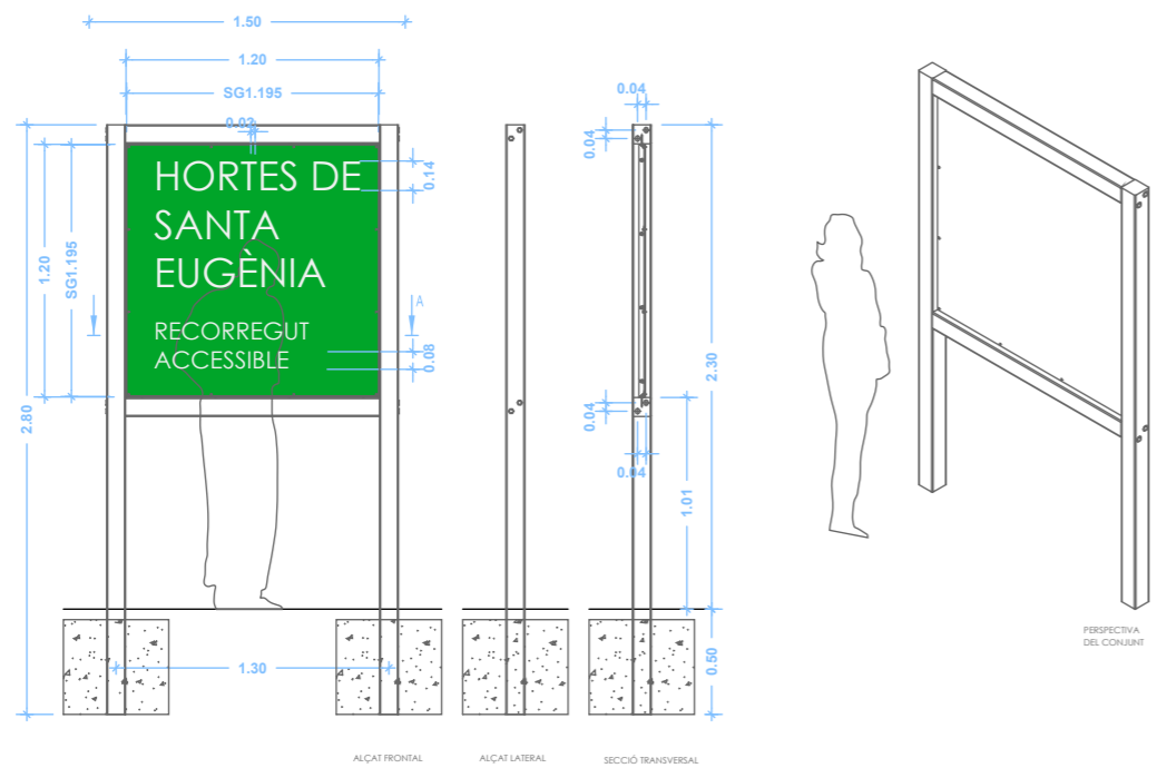
2.2.2.1.2 - Proposta S2 - Millora en la senyalització d'accés
