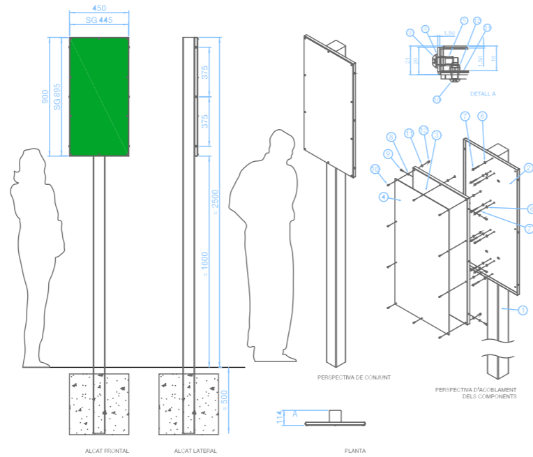
2.2.2.1.5 - Proposta S5 - Secció - Millora d'indicadors de Recorregut
