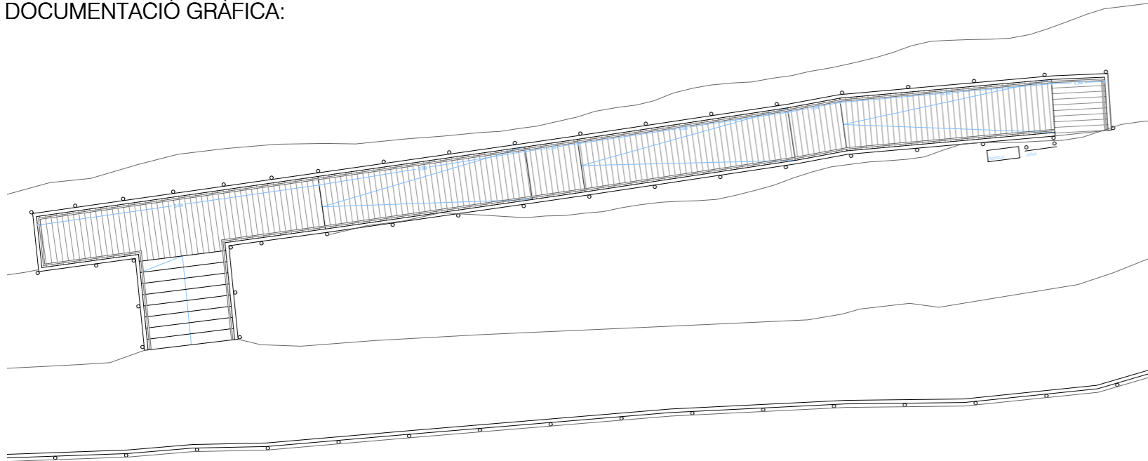
2.1.2.1.6 - Proposta A6 - Planta Rampa d'Accés amb Pendent Accessible
