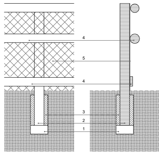
2.2.1.1.12 - Proposta C12 - Secció 1 : 25
