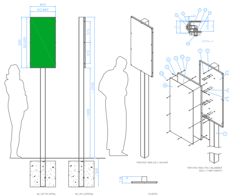
2.2.2.1.10 - Proposta S10 - Secció - Col·locació d'indicadors de recorregut
