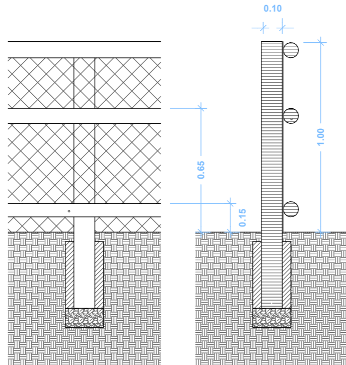
2.2.1.1.14 - Proposta C14 - Millora Protecció de Desnivell
