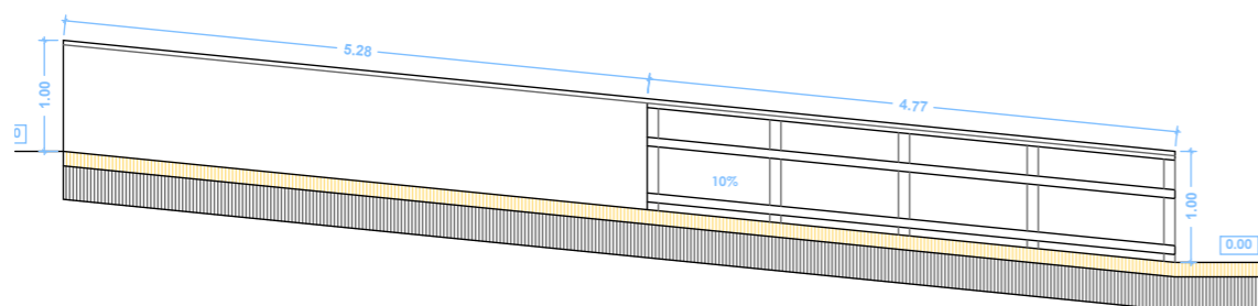
2.1.2.1.11 - Proposta A11 - Secció - Rampa d'Accés amb Pendent Accessible
